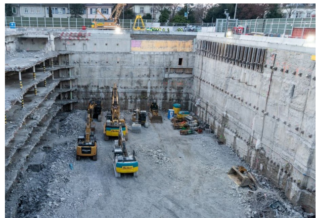
Basel – Roche Bau 74 41'000 Laufmeter Litzanker bis 40 Meter
